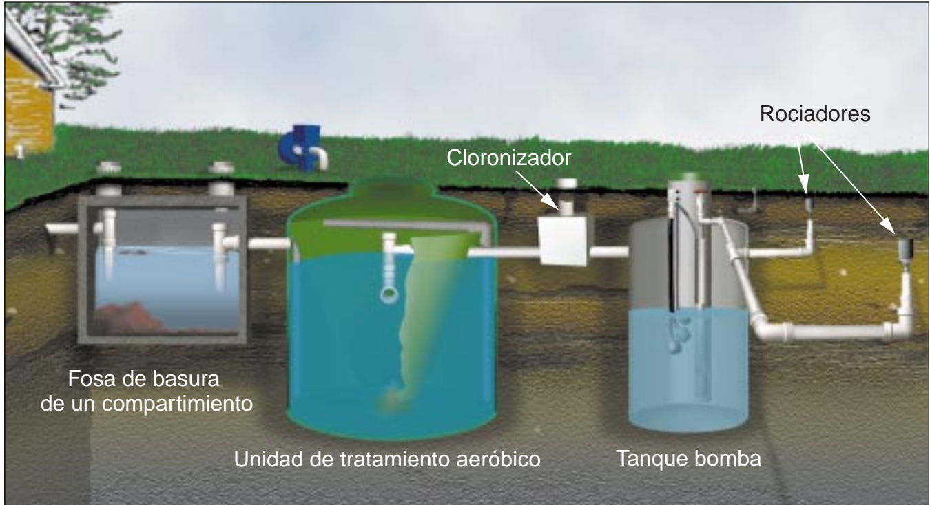
Figura 1: Un sistema individual para el tratameinto de agua negras con una unidad de tratamiento aeróbico.
