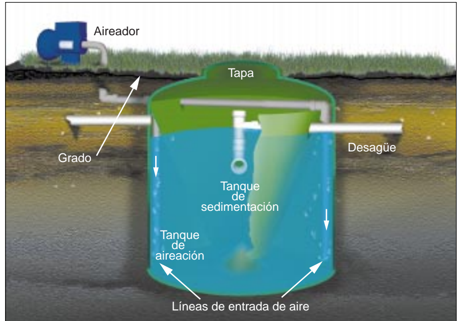
Figura 2: Una unidad de tratamiento aeróbico.
